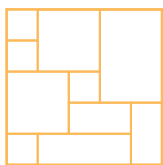
RÖMISCHER VERBAND Fliesen verschiedener Größen, ohne kreuzende Fugen
